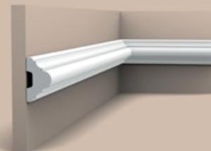
1 P4020 | P4020F 200 x 5 x 2,9 cm Purotouch ®
