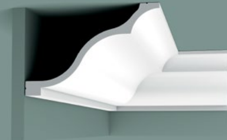
C337 200 x 17,2 x 25,6 cm Purotouch ®
