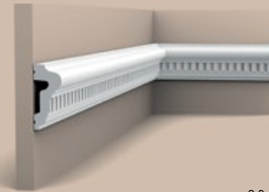
P6020 | P6020F 200 x 6,4 x 2,8 cm Purotouch ®
