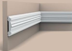
P9020 | P9020F 200 x 9,6 x 2,1 cm Purotouch ®
