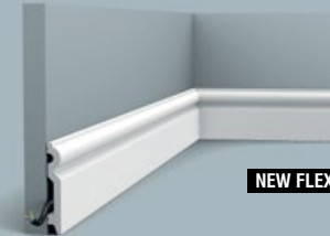
SX137 | SX137F 200 x 9,9 x 1,5 cm Duropolymer ®
